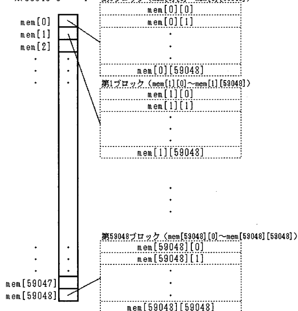
図 1 Malbolge20 のメモリイメージ図
